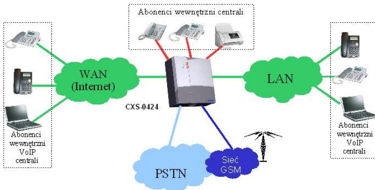
Ilustracja 1.6.: Centrala CXS-0424.WM z funkcjonalnością VoIP
