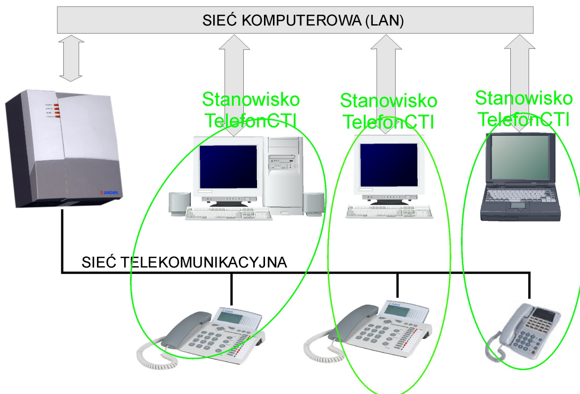
Ilustracja 1.2.: Współpraca centrali CXS-0424.WM z aplikacjami CTI
