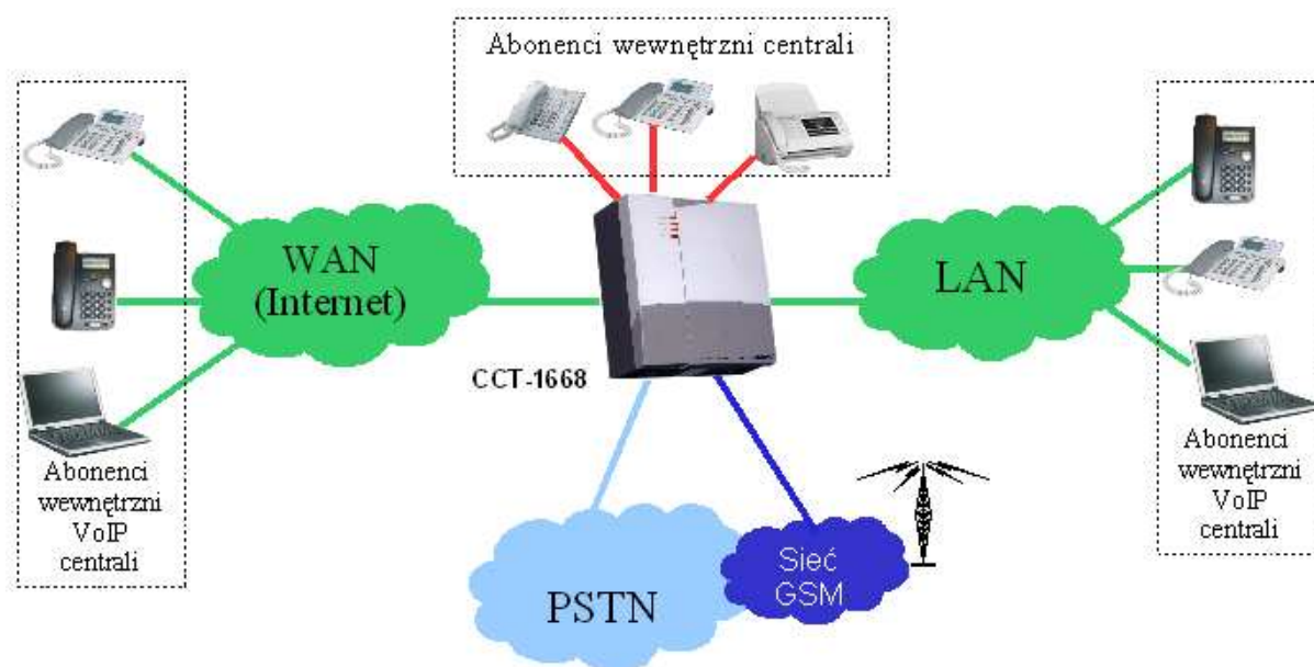
Ilustracja 1.6.: Centrala CCT-1668.S z funkcjonalnością VoIP
