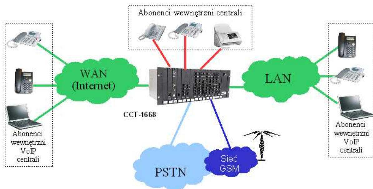
Ilustracja 1.6.: Centrala CCT-1668.EU z funkcjonalnością VoIP
